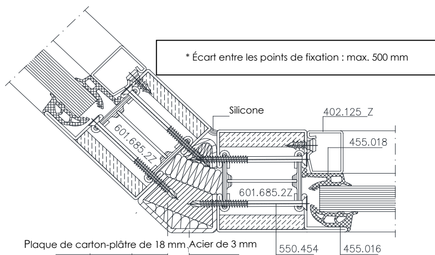
Coupe 7.1.3 – Janisol 2
