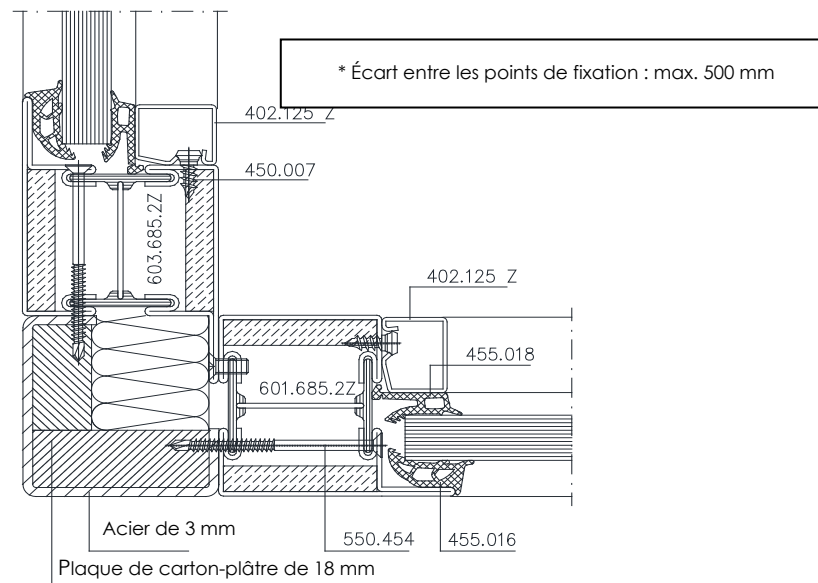
Coupe 7.1.3 – Janisol 2
