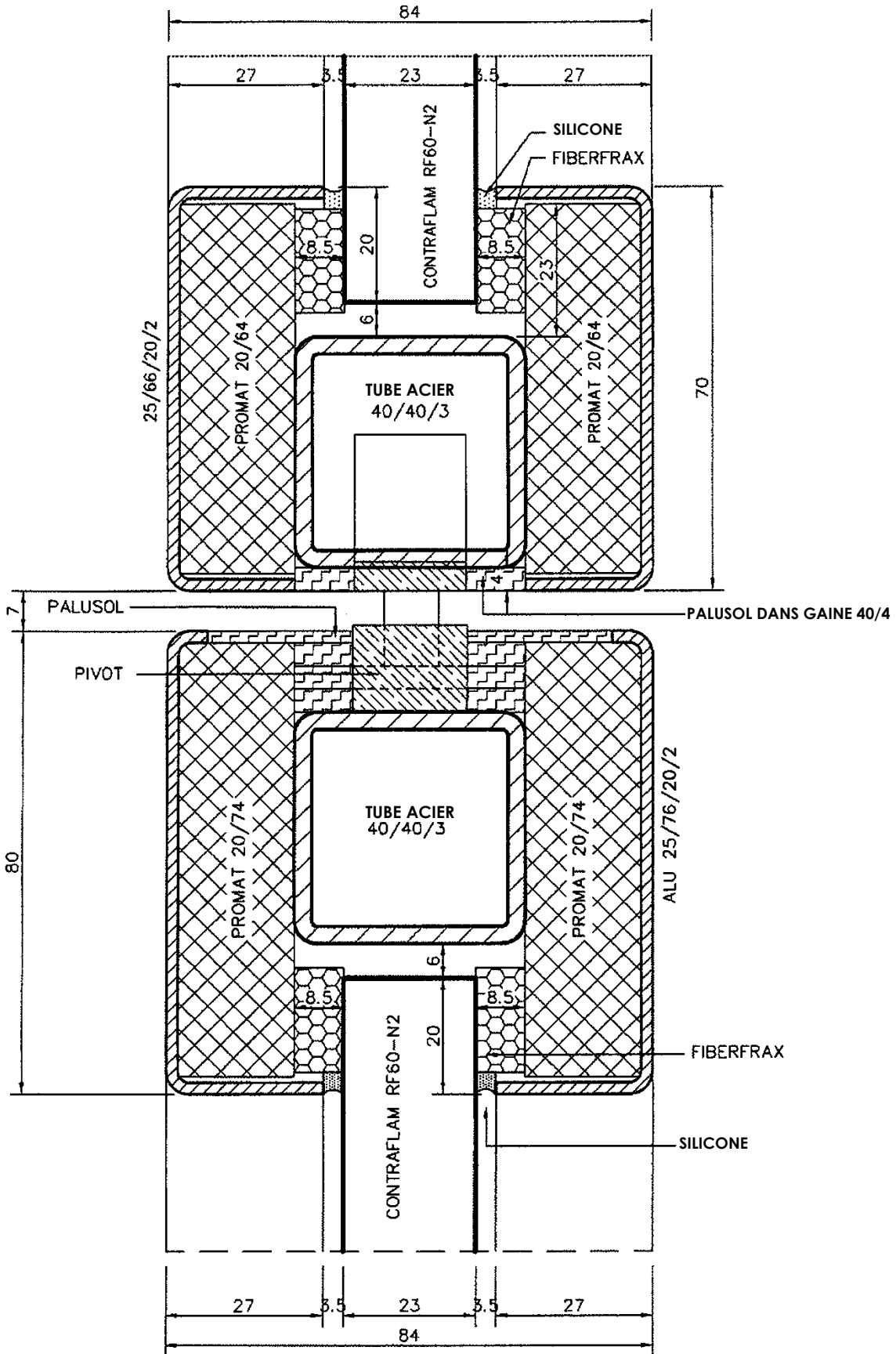
Coupe 8 : Raccord vantail-imposte vitrée
