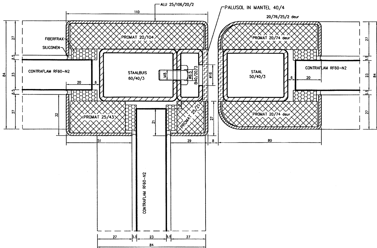
Figuur 2: Afmetingen Contraflam 60 N2
