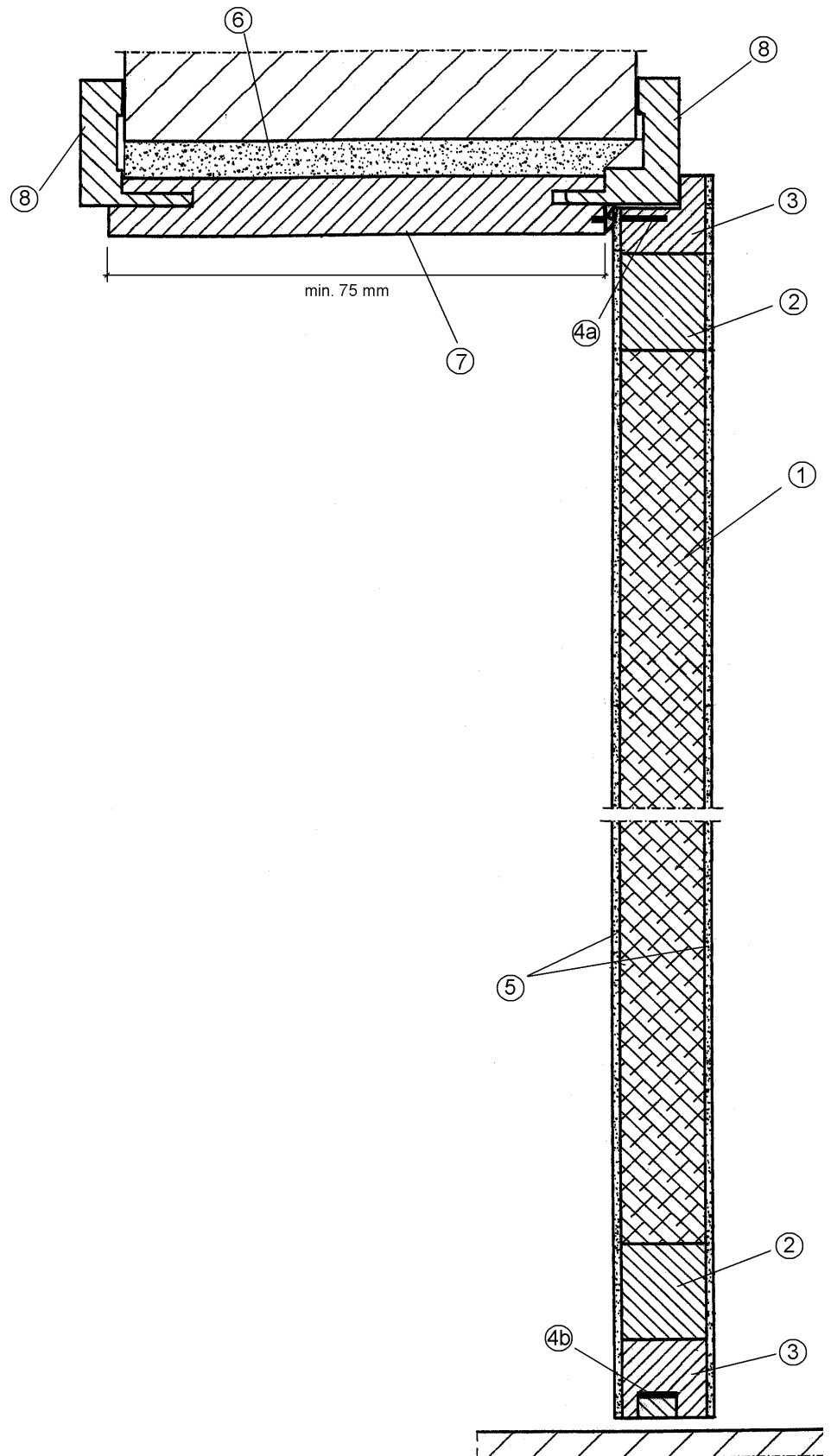
Figuur 1a: Verticale doorsnede LIBERT BF 1
