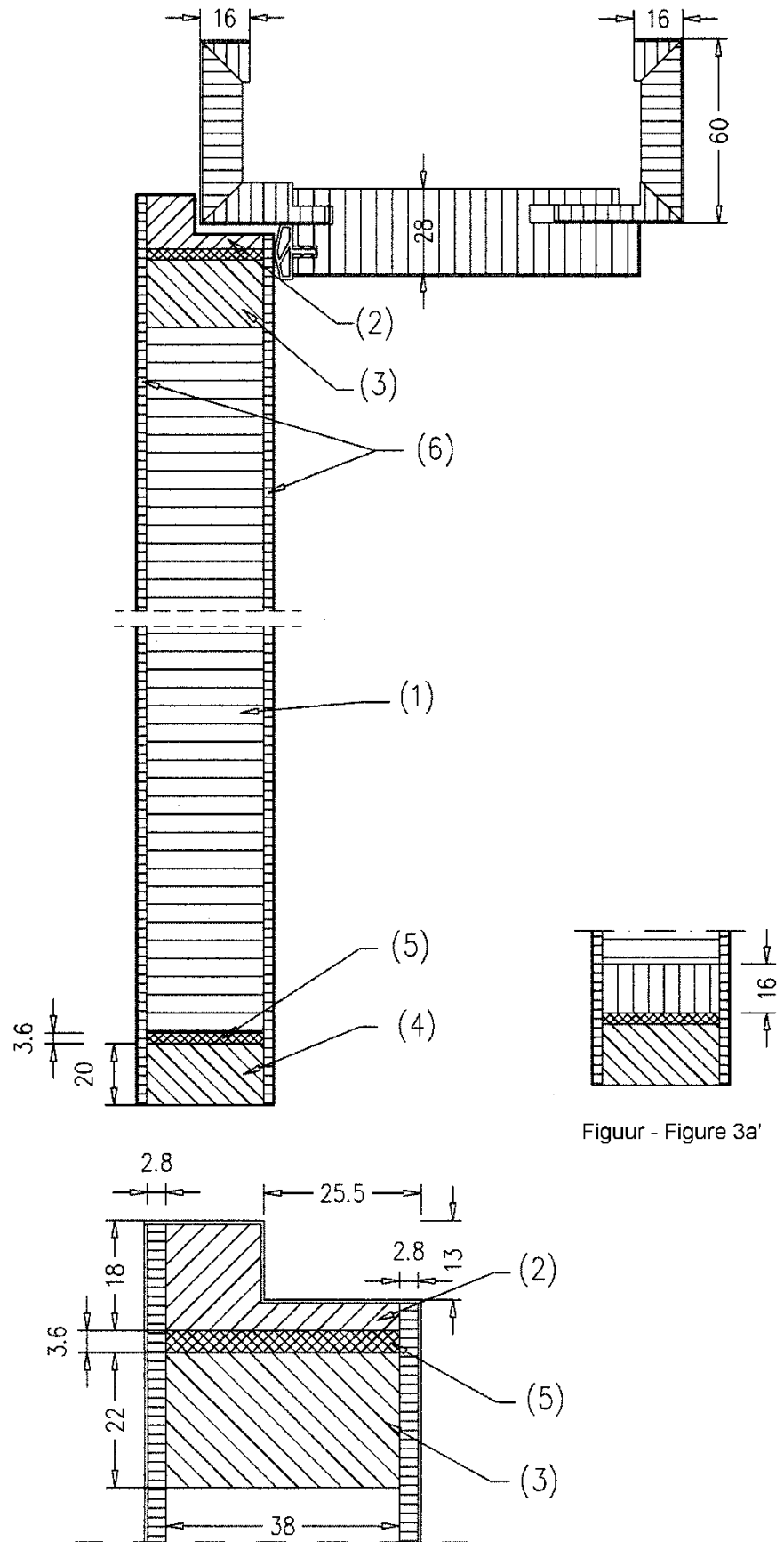
Figuur 3a: Verticale doorsnede LIBERT BF 4
