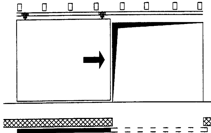
Figure 1a : Porte coulissante simple
