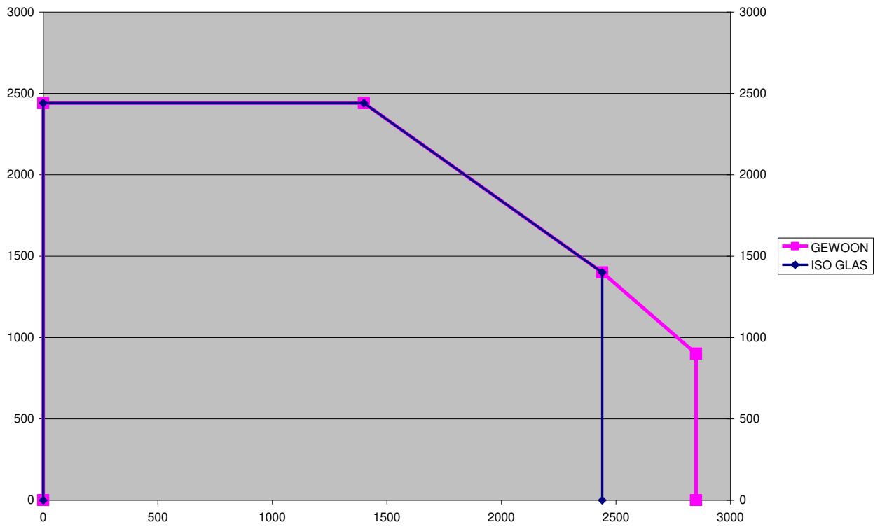
Figure 7 : Paroi vitrée : dimensions maximales des vitrages
