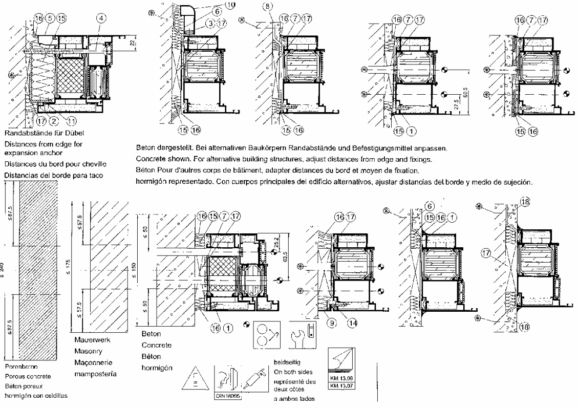
Figur 8a: Wandaansluiting
