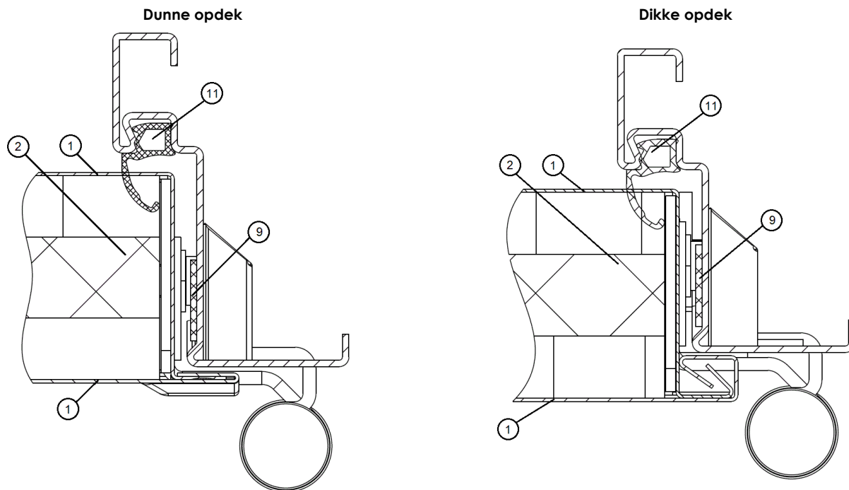
Fig. 6 Details scharnierzijde
