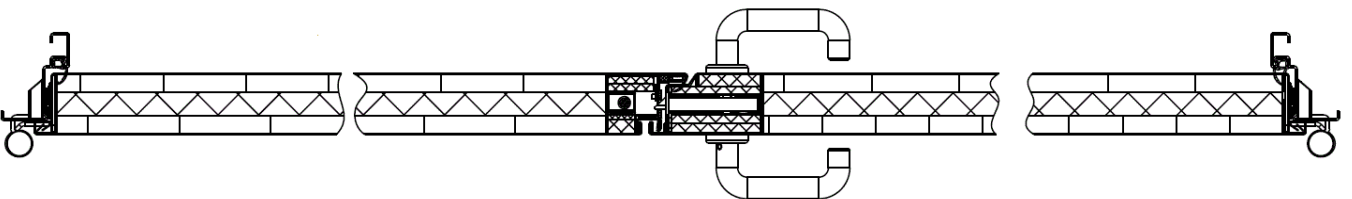
Fig. 4 Coupes horizontales
